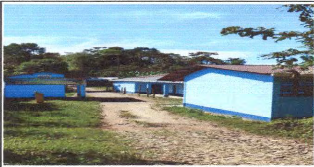
Foto 7: mantenimiento de lamina (cepillado y pintado)
